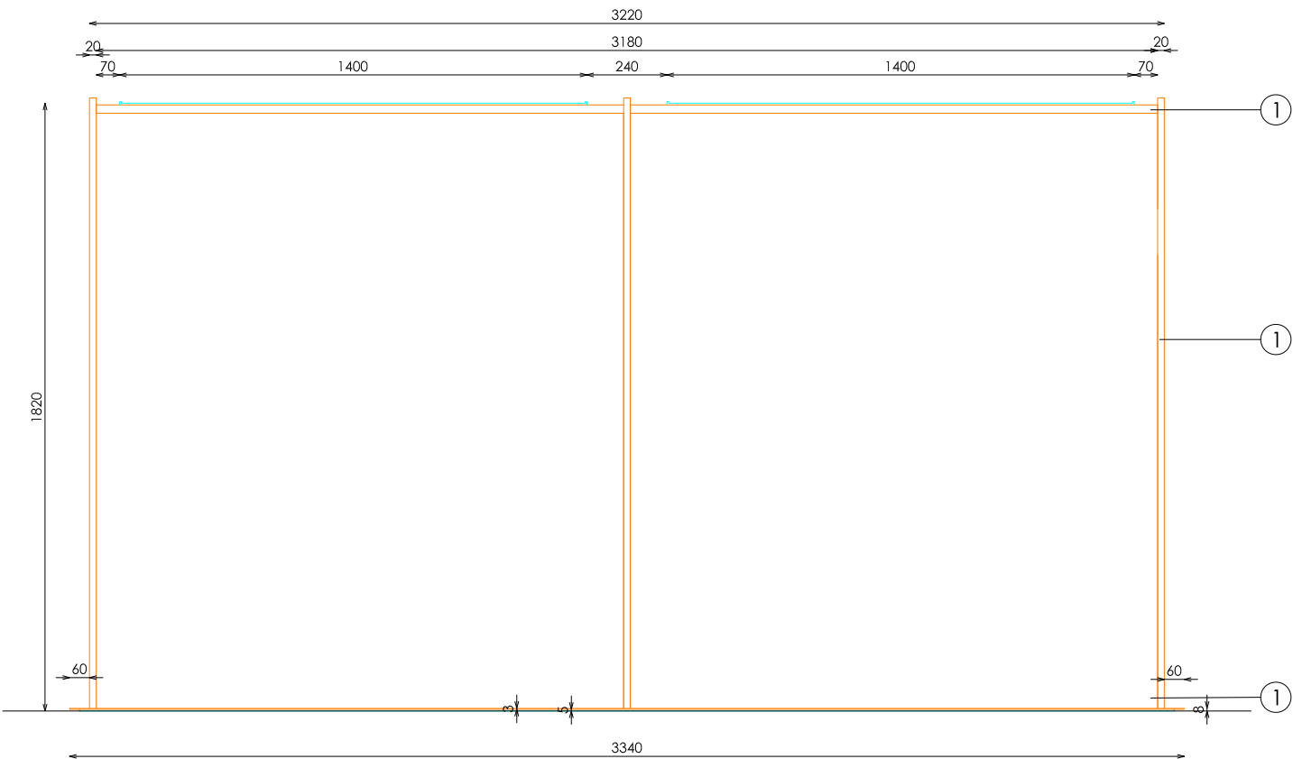
ALZADO SECCIONADO
