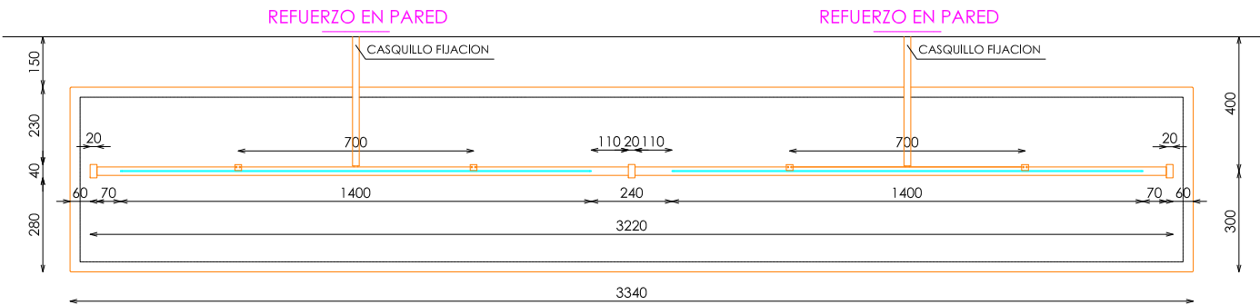
PLANTA
