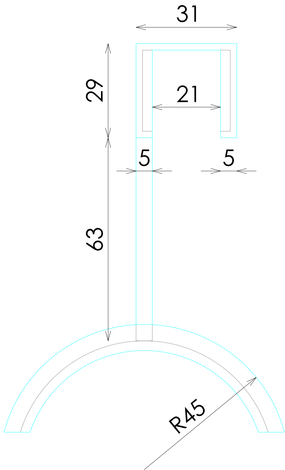
ALZADO
