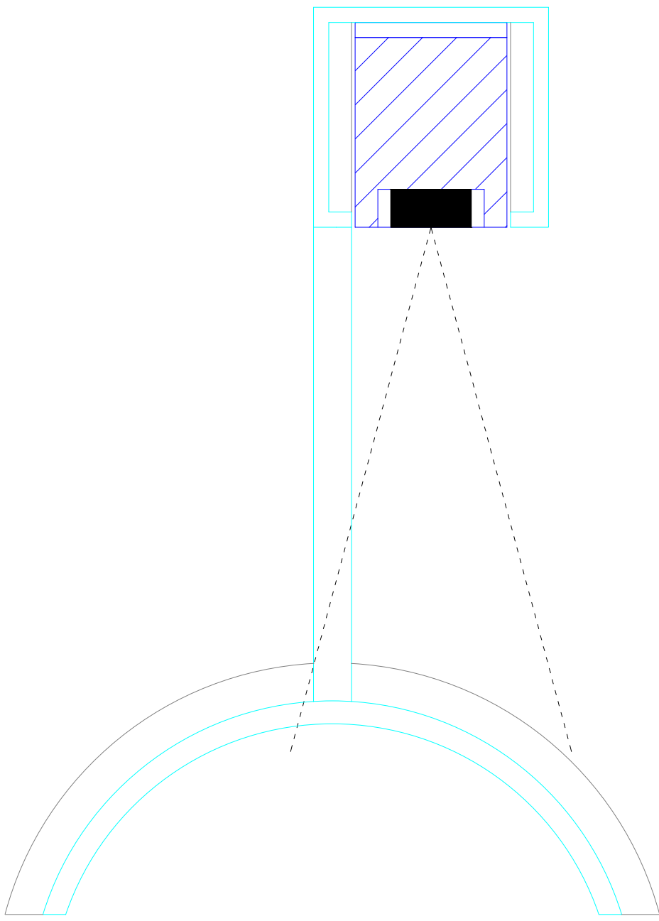
SECCION MONTAJE BARRA 20x25
