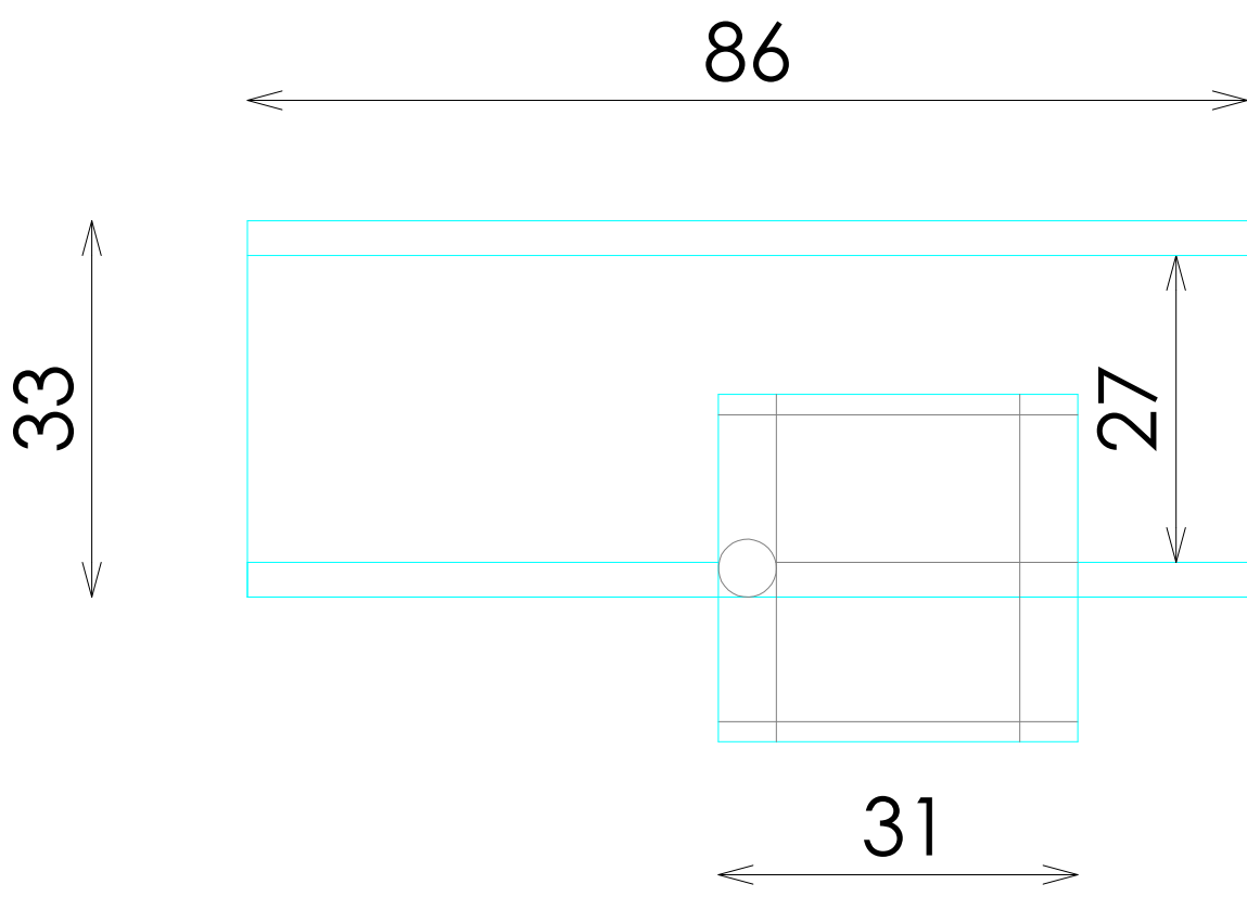
PLANTA
