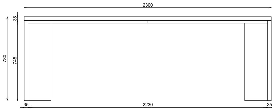
ALZADO POSTERIOR
