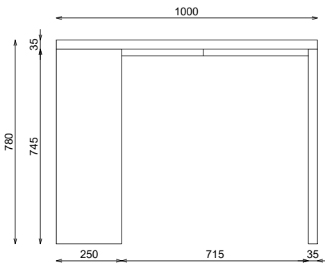
ALZADO LATERAL
