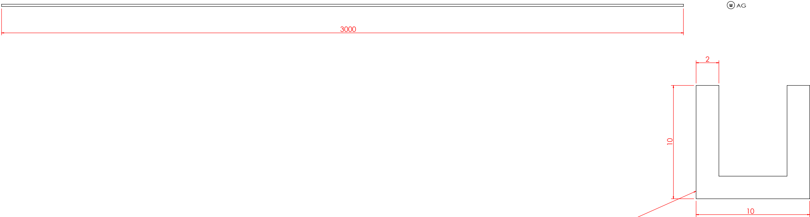
局部视图 AG 比例 5 : 1
