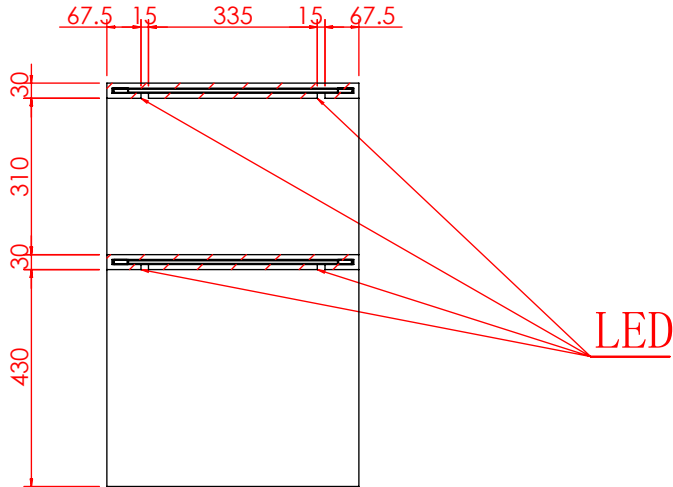
剖面 AG-AG
