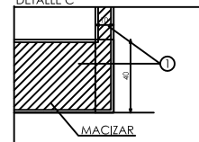
DETALLE C
