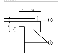
DETALLE C
