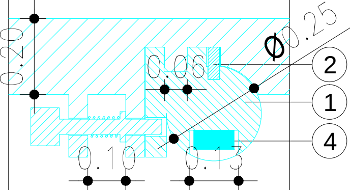
DETALLE ANCLAJE FRONTALES EXTRAIBLES
