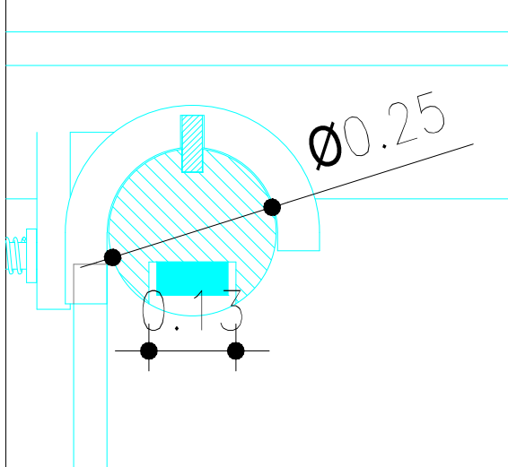
DETALLE BARRA ANCLAJE FRONTALES
