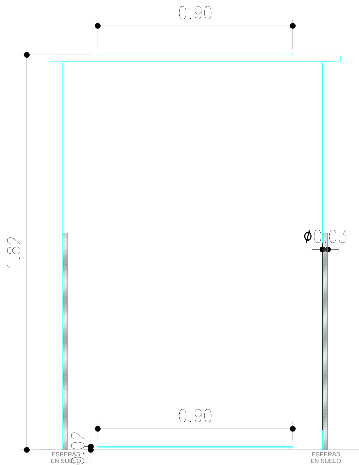
ALZADO FRONTAL
