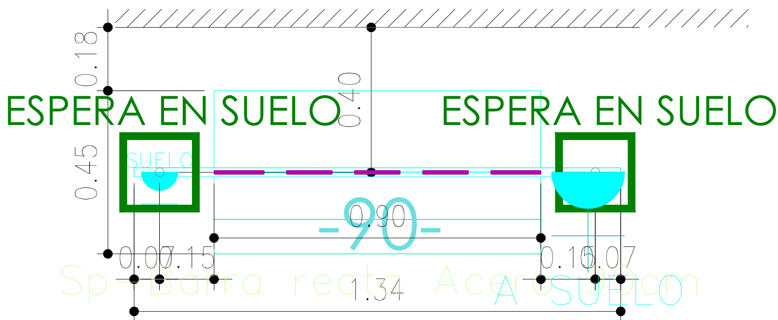
PLANTA
