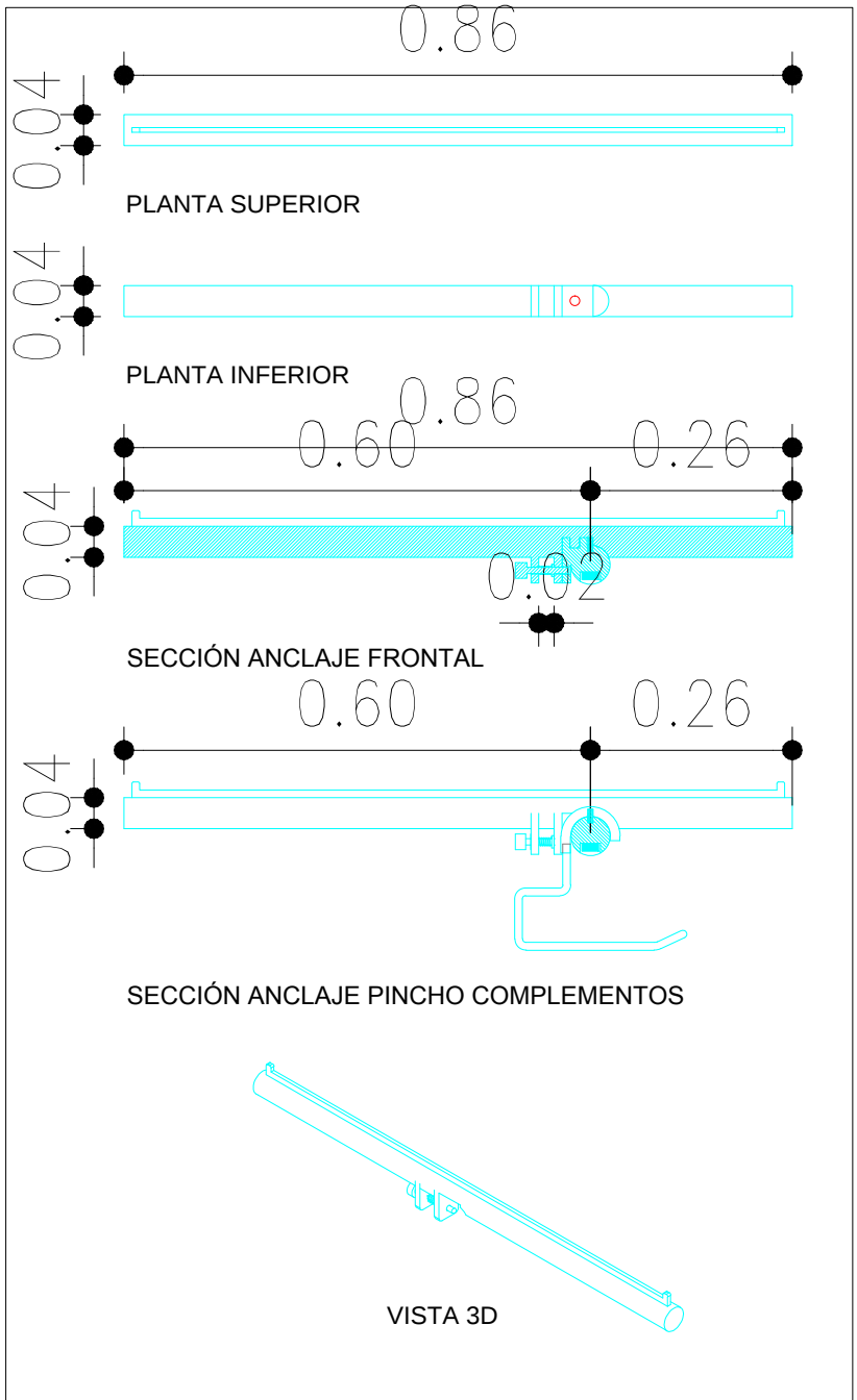
FRONTAL EXTRAIBLE
