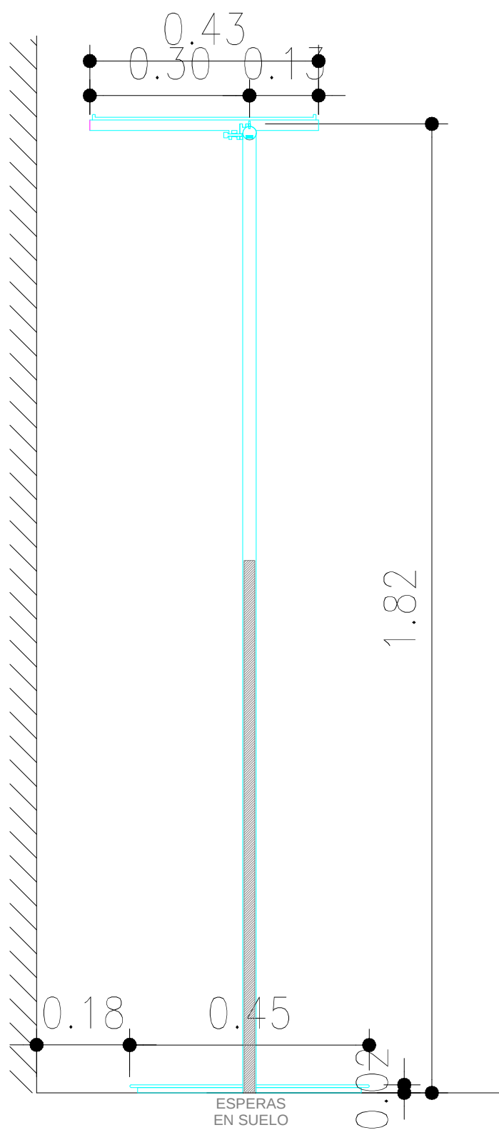
SECCIÓN
