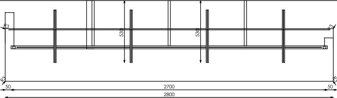
PLANTA
