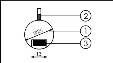
DETALLE BARRA+ILUMINACION
