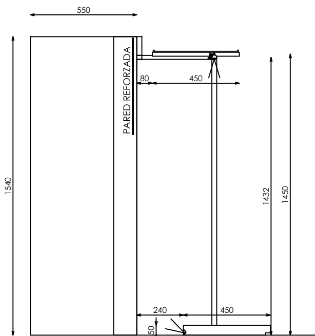
SECCIÓN
