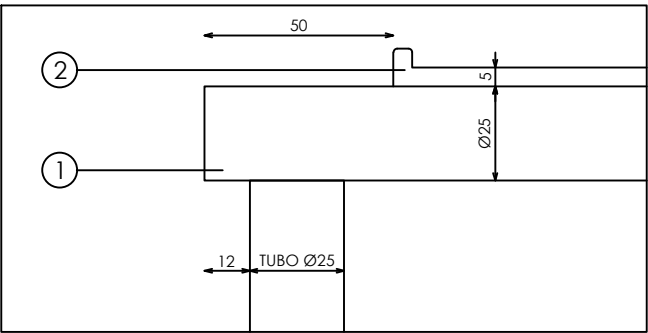
DETALLE FRONTALES EXTRAIBLES
