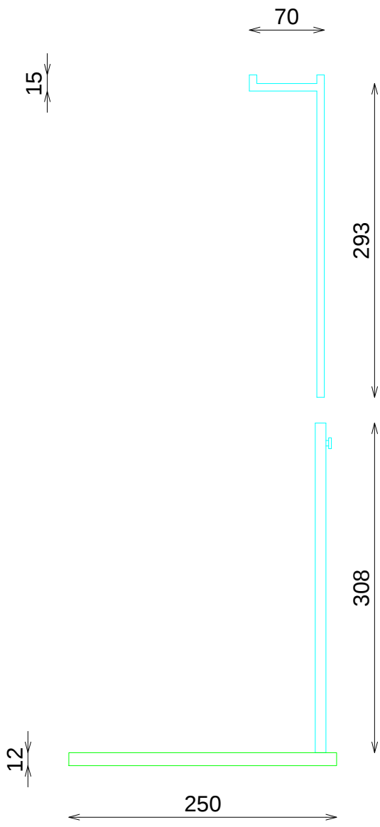
ALZADO B
