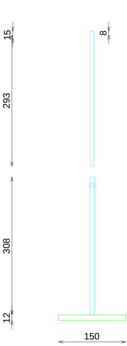
ALZADO C
