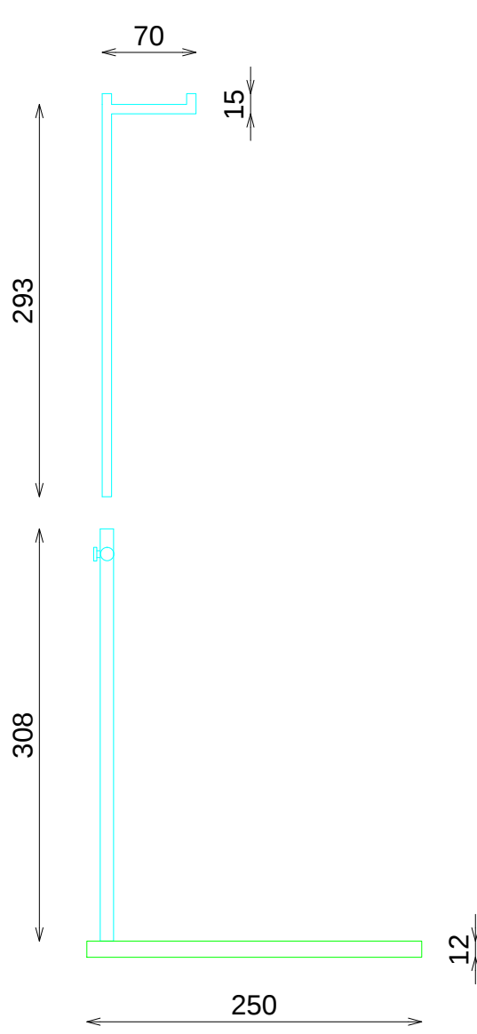
ALZADO D
