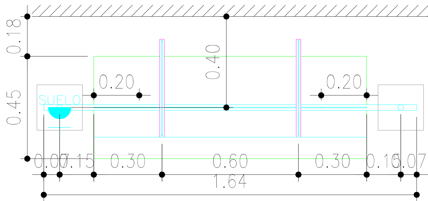
PLANTA
