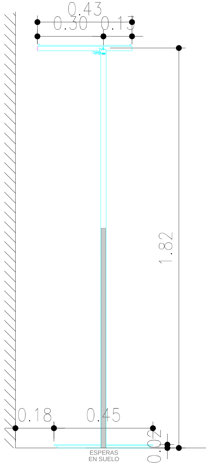
SECCIÓN
