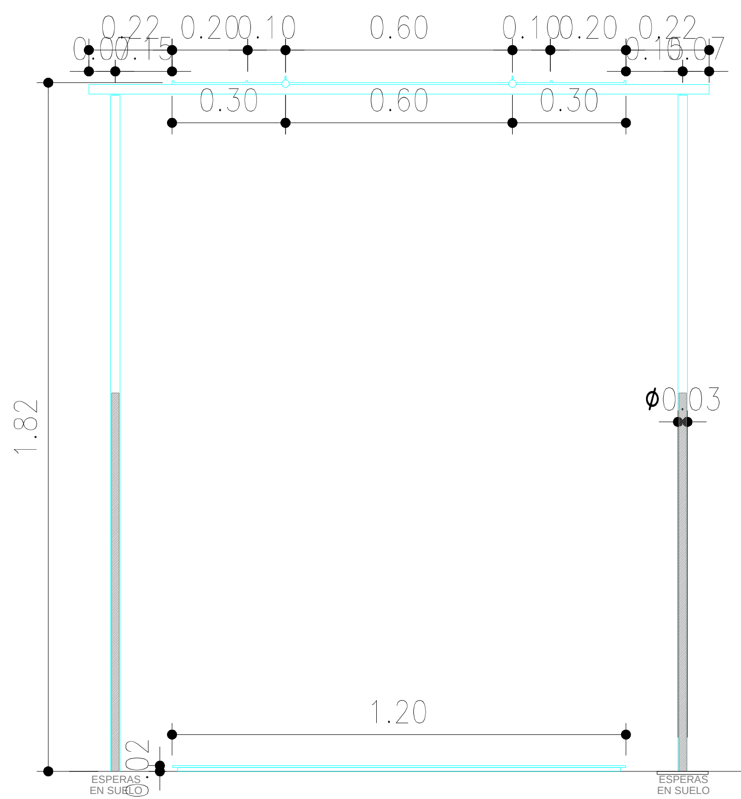
ALZADO FRONTAL
