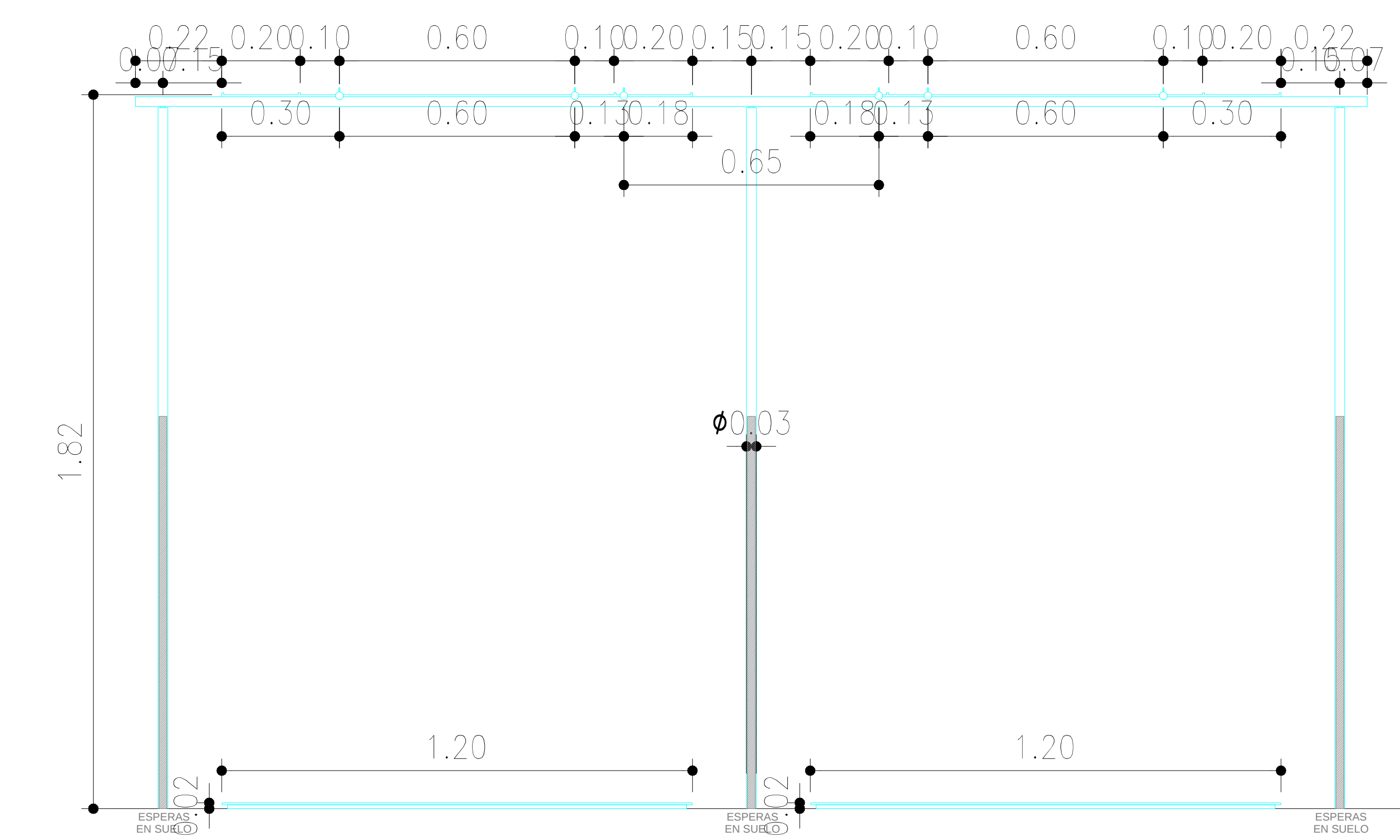
ALZADO FRONTAL
