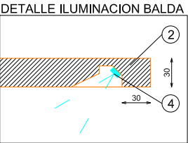
DETALLE ILUMINACION BALDA
