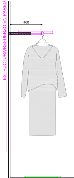
SECCION
