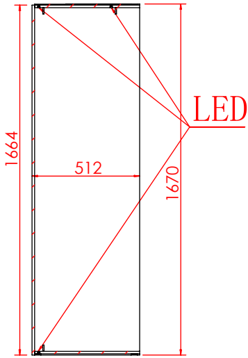
剖面 AG-AG
