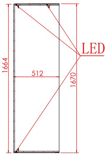
剖面 AG-AG
