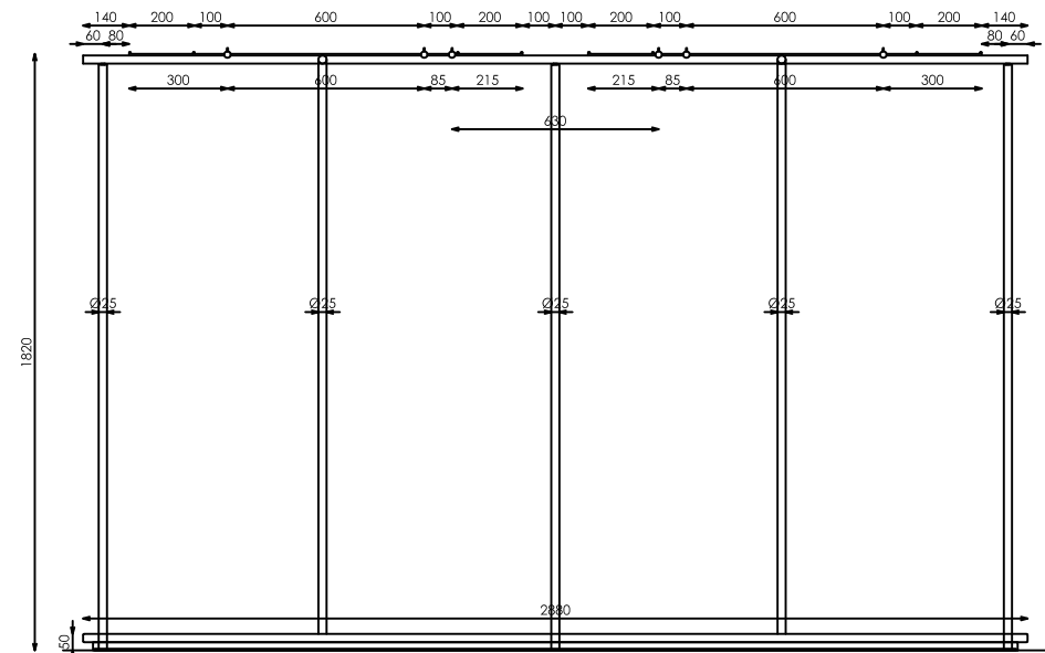
ALZADO FRONTAL
