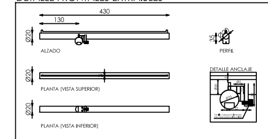
DETALLE FRONTALES EXTRAIBLES
