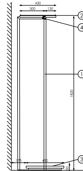
SECCIÓN
