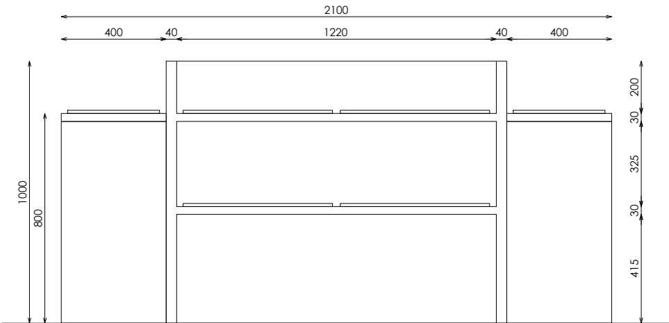
ALZADO FRONTAL
