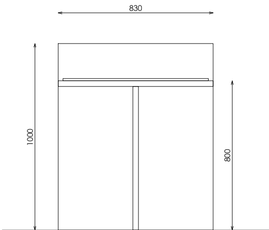
ALZADO LATERAL
