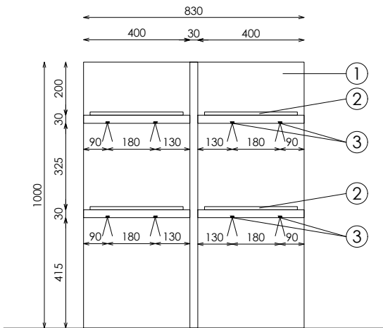
SECCION TRANSVERSAL
