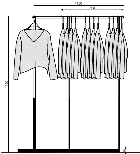
ALZADO FRONTAL
