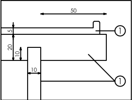
DETALLE C
