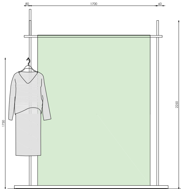
ALZADO DERECHO
