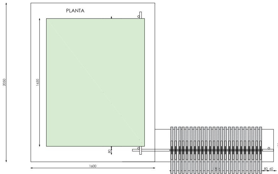
PLANTA
