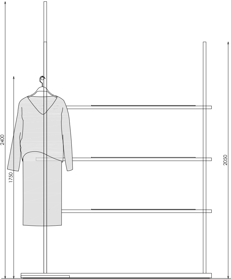
ALZADO DERECHA
