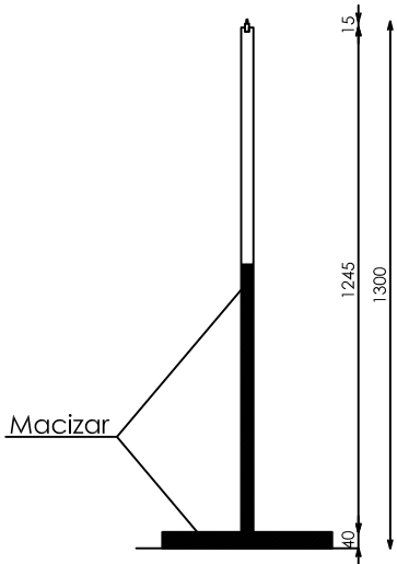
SECCIÓN
