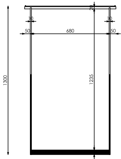
ALZADO
