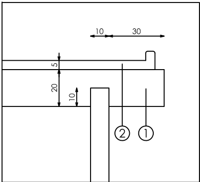
DETALLE C
