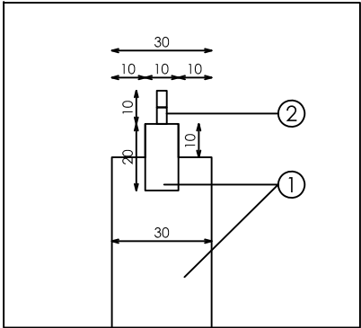
DETALLE B
