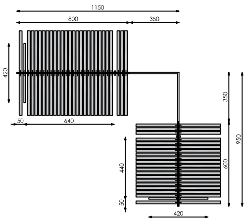
PLANTA
