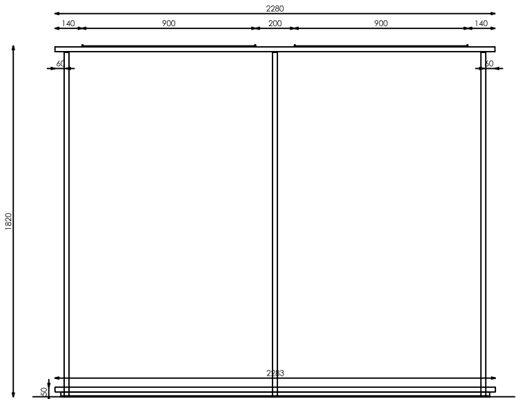
ALZADO
