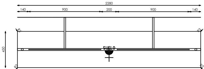
PLANTA
