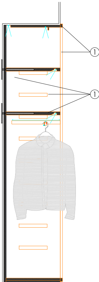
SECCIÓN BARRA BAJA
