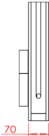
局部视图 F
