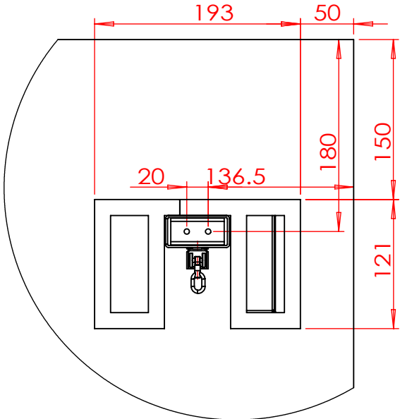
局部视图 G
