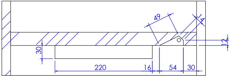
局部视图 AI 比例 1 : 5
