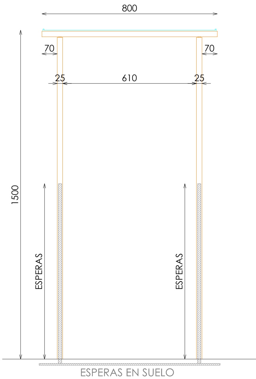
ALZADO
