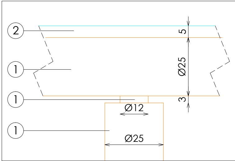
DETALLE B
