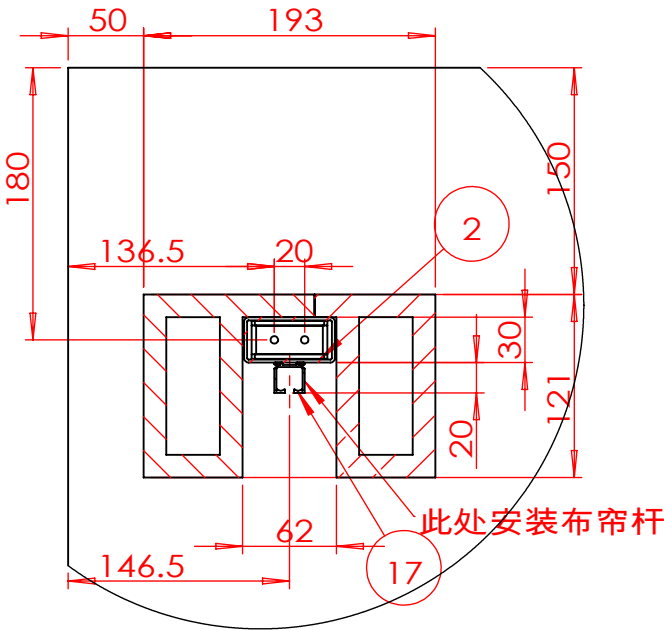
局部视图 D
