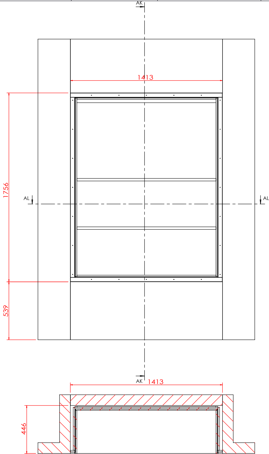
剖面 AL-AL
