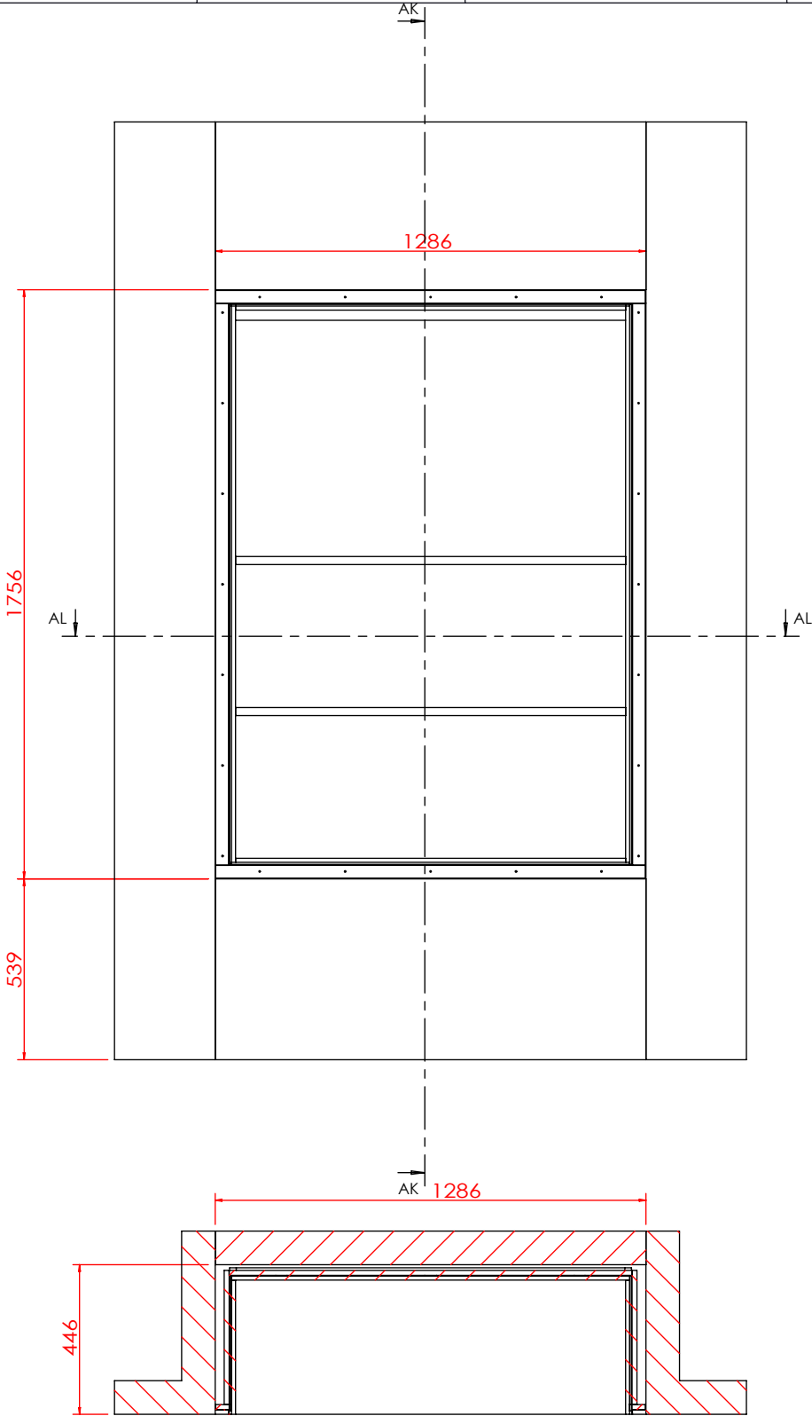
剖面 AL-AL
