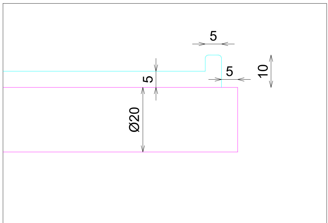
DETALLE B
