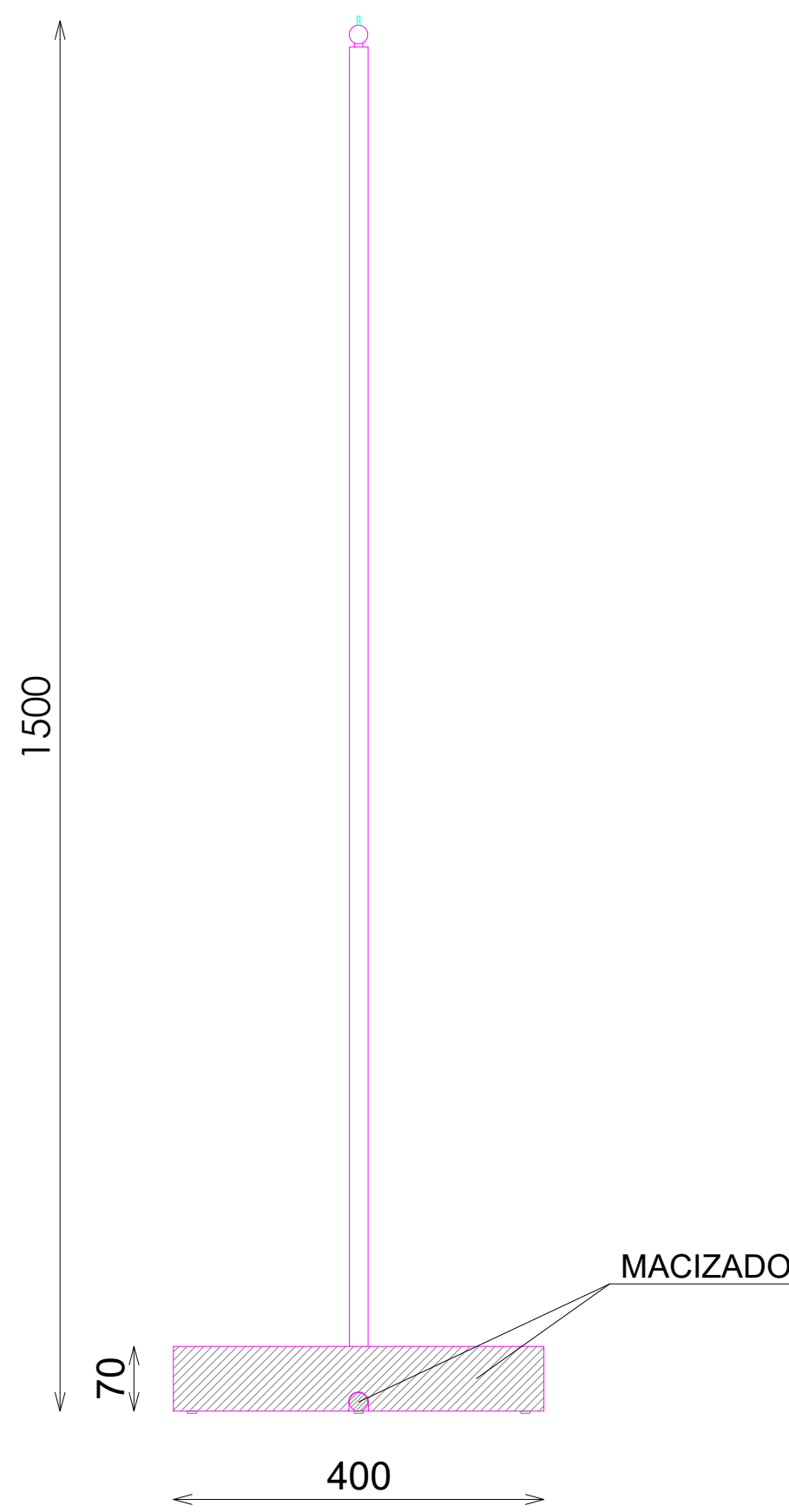
PERFIL
