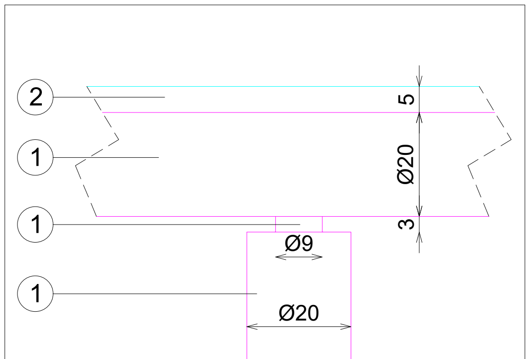
DETALLE A
