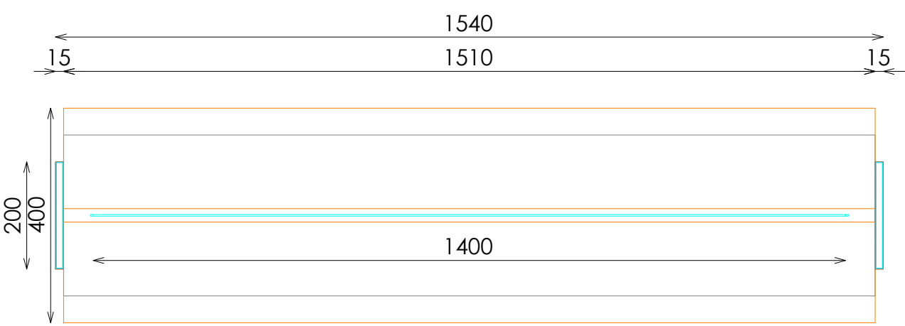
PLANTA SECCIONADA
