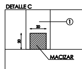
DETALLE C
