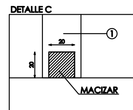
DETALLE C
