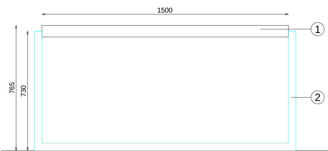
ALZADO LATERAL
