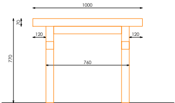
ALZADO LATERAL
