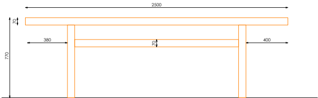
ALZADO FRONTAL
