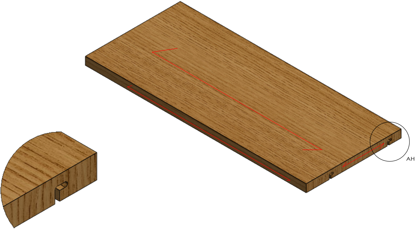
局部视图 AH 比例 1 : 2
