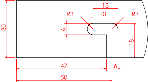
局部视图 AG 比例 1 : 1
