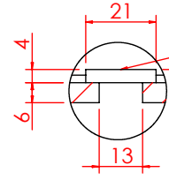
局部视图 AI 比例 1:2
