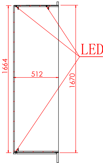
剖面 AG-AG
