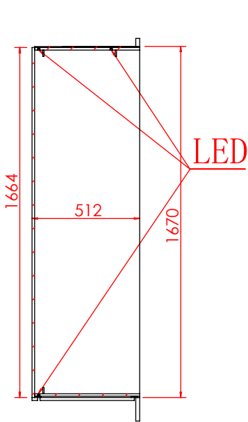
剖面 AG-AG
