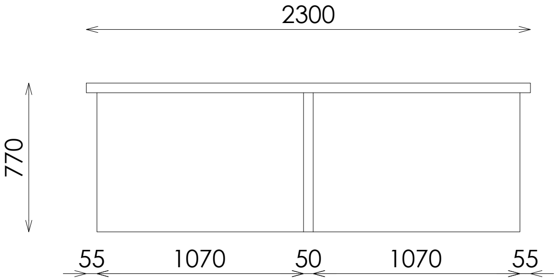
ALZADO FRONTAL
