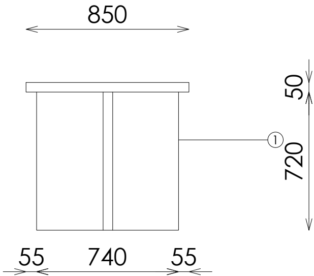
ALZADO IZQUIERDA
