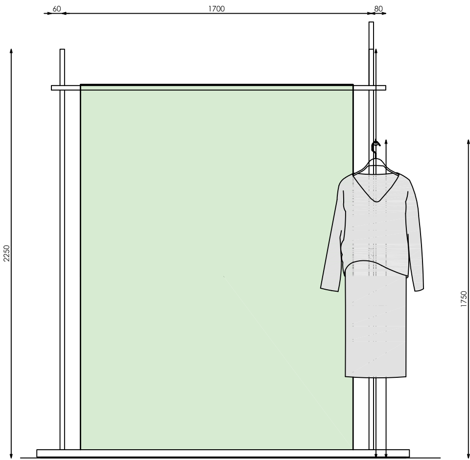
ALZADO DERECHO
