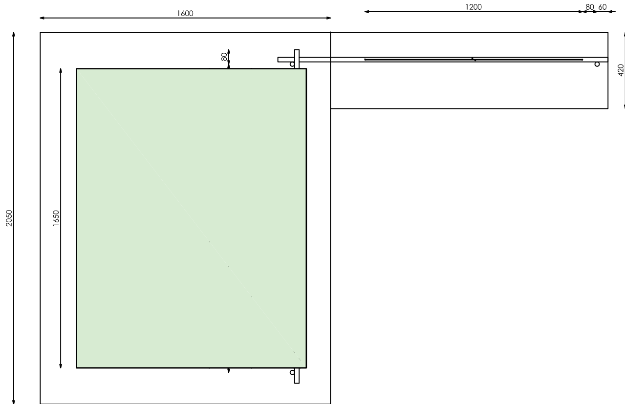
PLANTA
