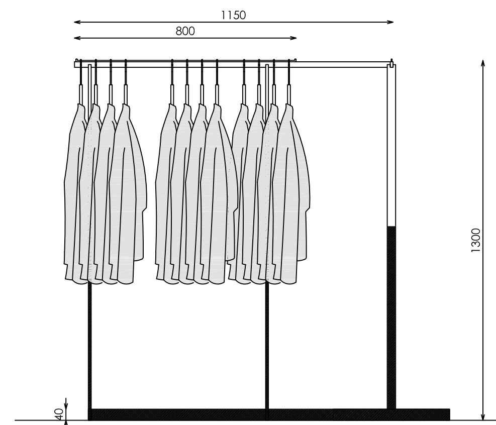
ALZADO FRONTAL
