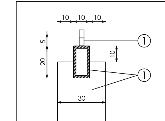
DETALLE B
