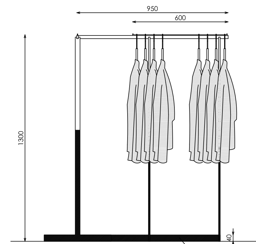
ALZADO LATERAL
