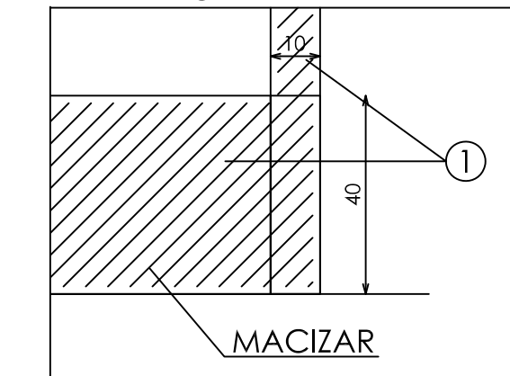
DETALLE C
