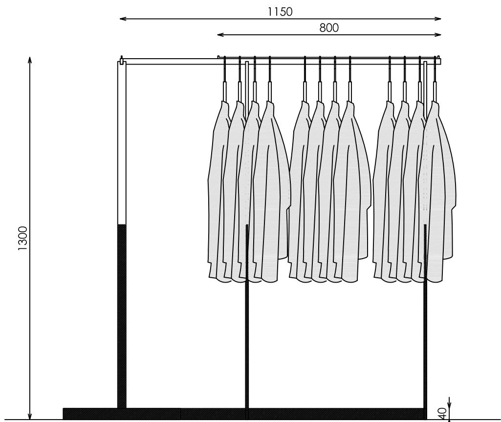
ALZADO FRONTAL
