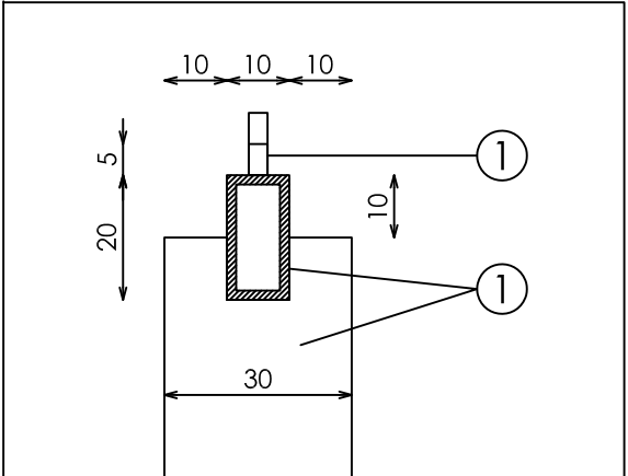
DETALLE B
