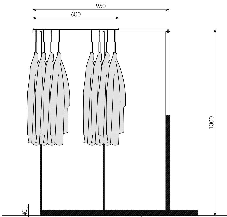
ALZADO LATERAL
