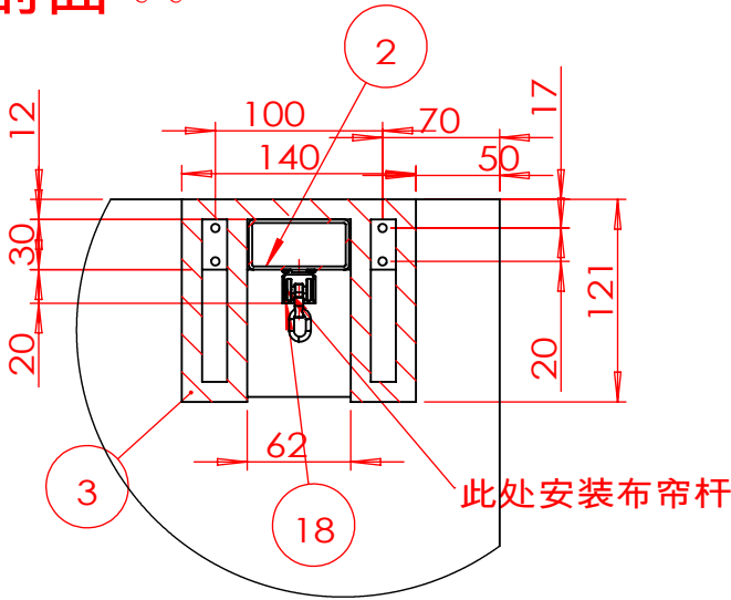
剖面 C-C
