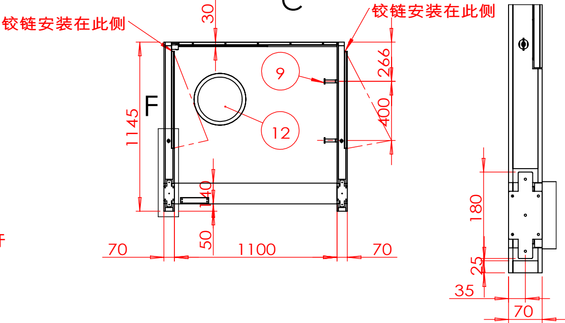
局部视图 F
