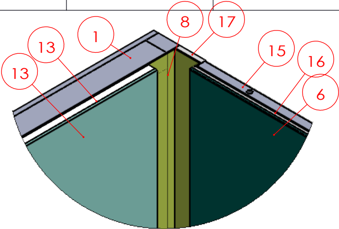
局部视图 E 比例 1 : 5
