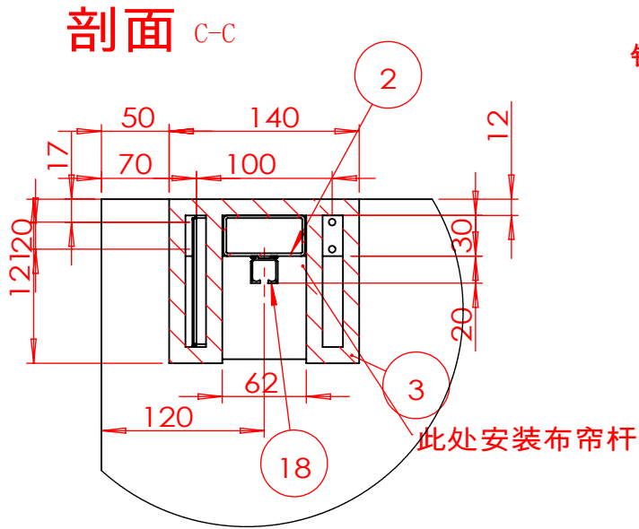
局部视图 D 比例 1 : 5
