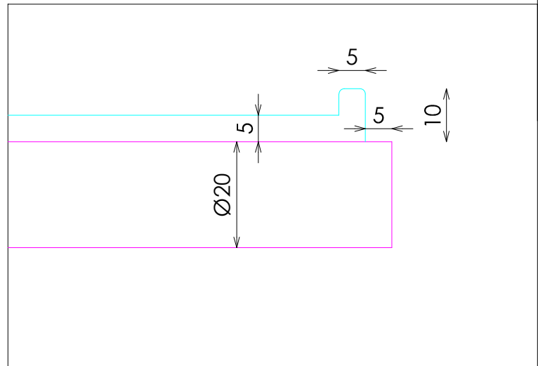
DETALLE C
