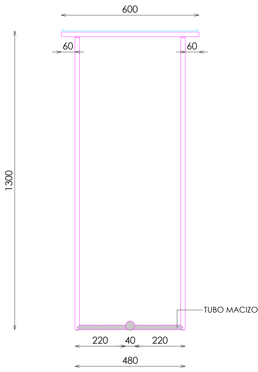
ESTRUCTURA
