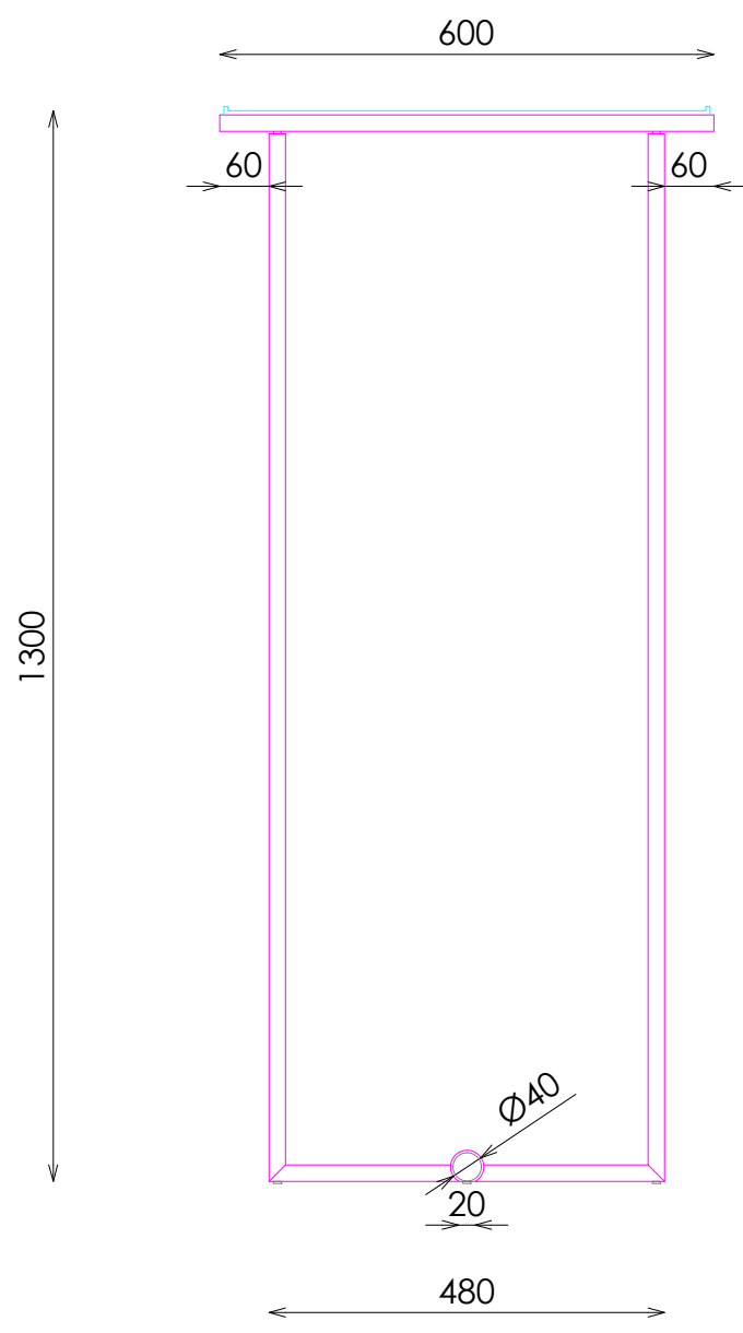
ALZADO
