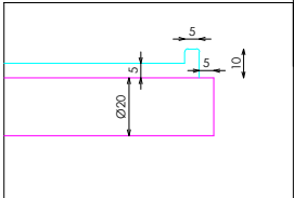
DETALLE C
