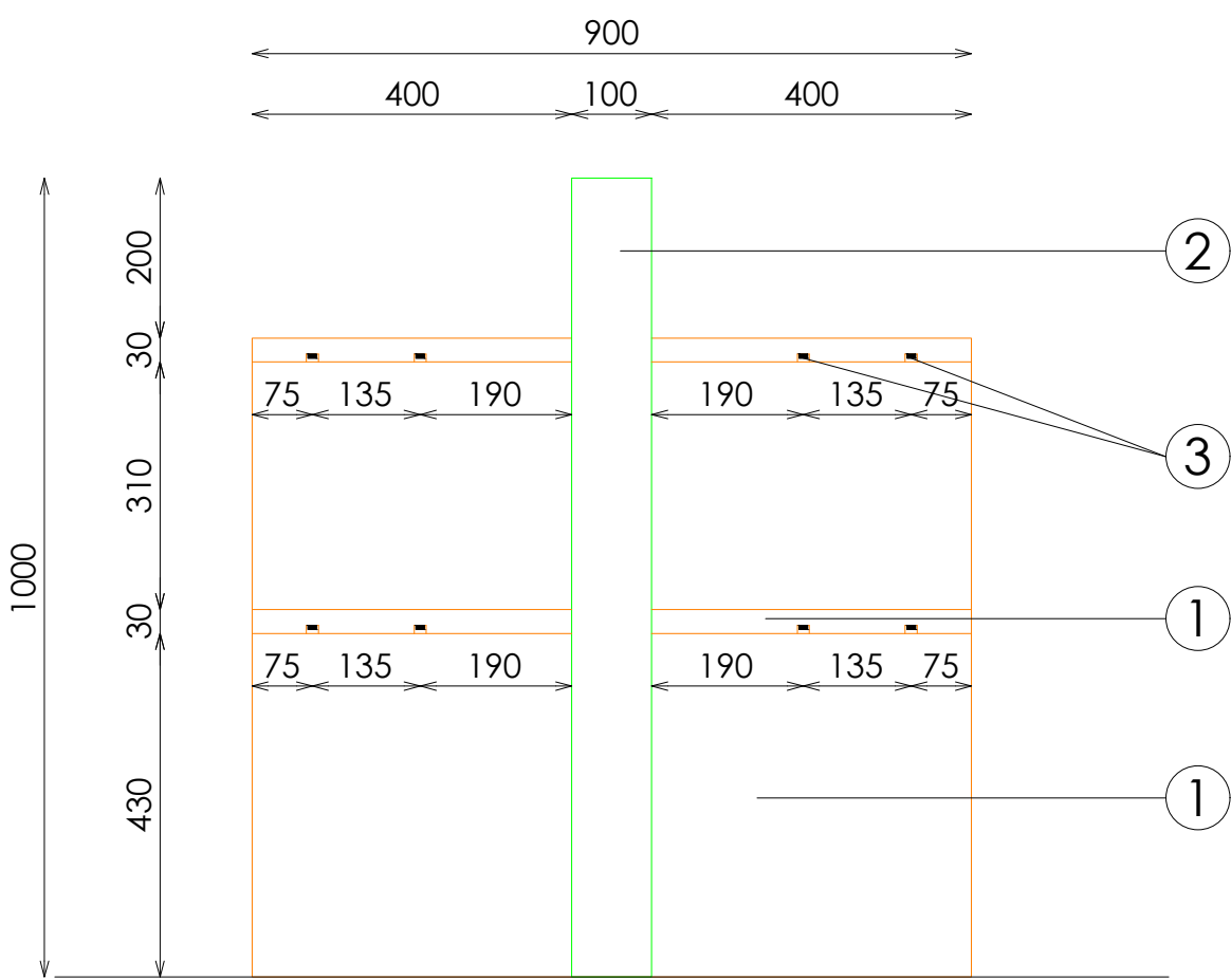
SECCION
