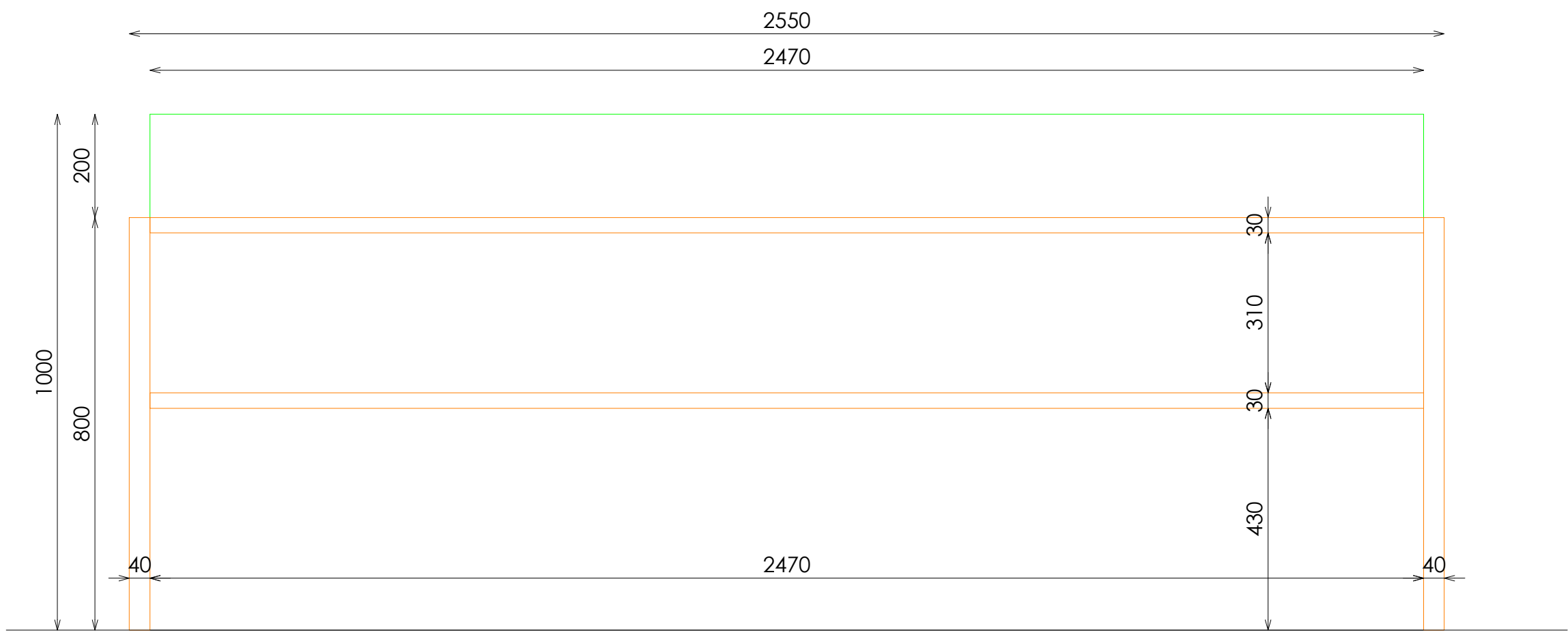
ALZADO FRONTAL
