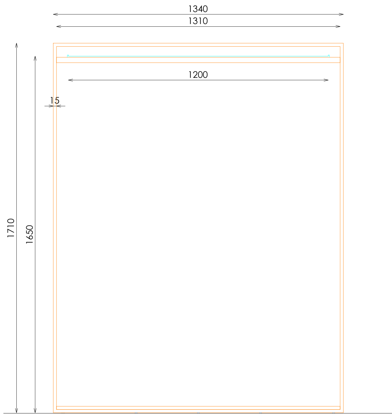
ALZADO
