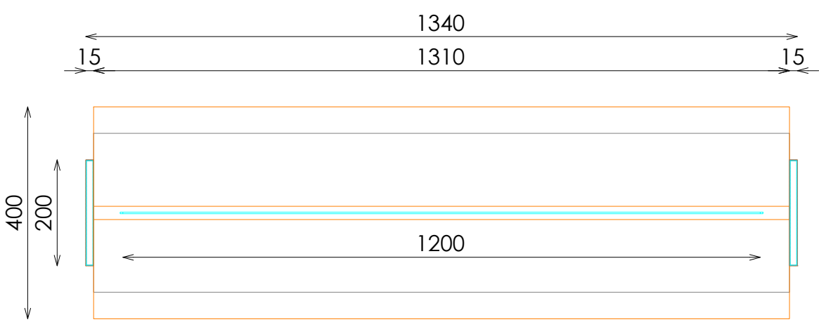
PLANTA SECCIONADA
