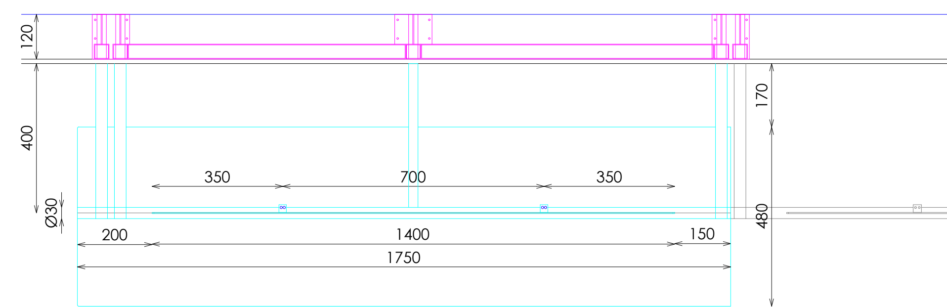
PLANTA
