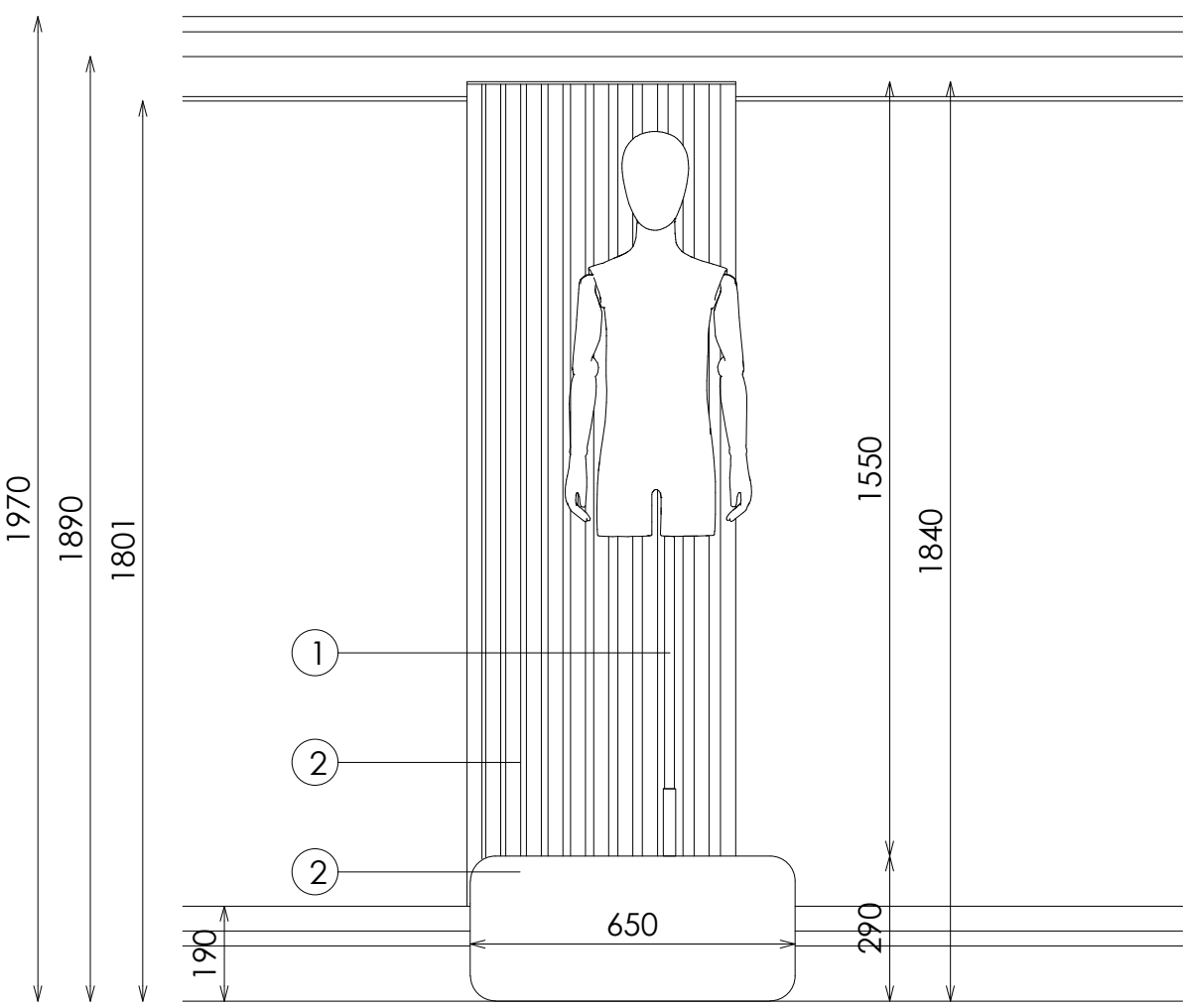
ALZADO FRONTAL
