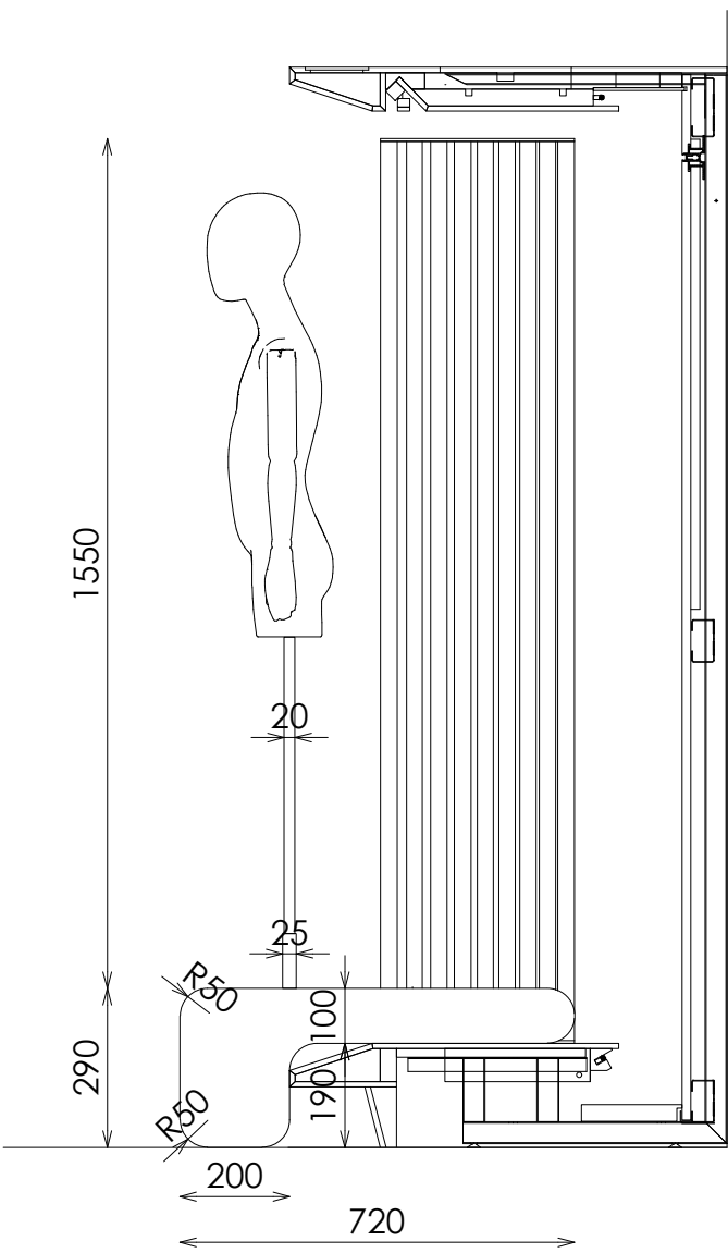
ALZADO LATERAL DERECHO
