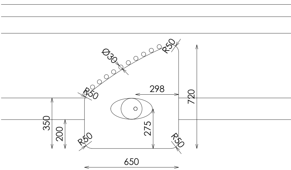
PLANTA
